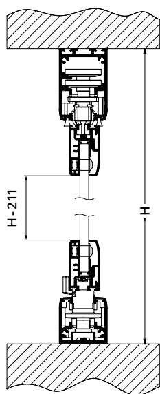
Fara profil telescopic superior, profil inferior standard
