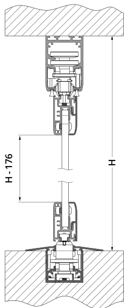
Fara profil telescopic superior, profil inferior incorporat
