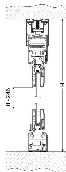
Cu profil telescopic superior, profil inferior standard
