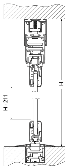
Cu profil telescopic superior, profil inferior incorporat
