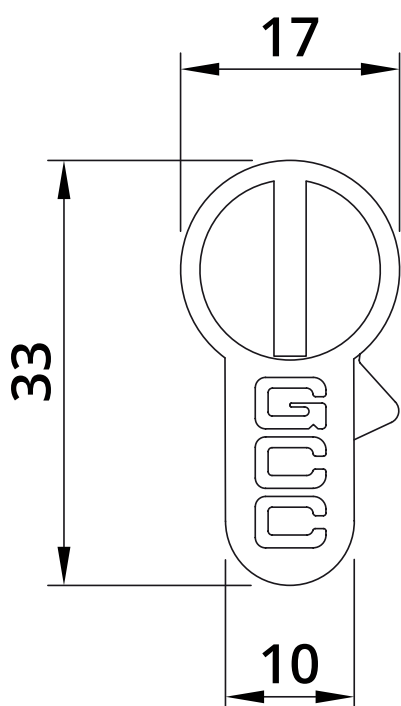
Cilindru baie broasca usa sticla 8-10 mm - dimensiuni de gabarit si constructive
